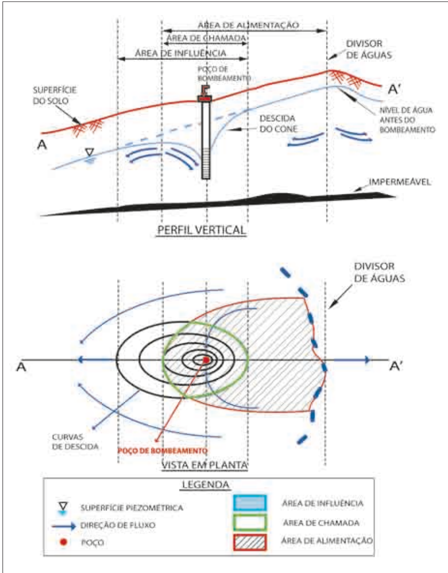
Figura B. Zona de Chamada de um poço em funcionamento (Navarrete & García 2003)
