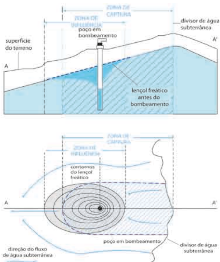
FIGURA 1. Zona de captura ou de contribuição de um poço em funcionamento (Fonte: Foster et al. 2006)
