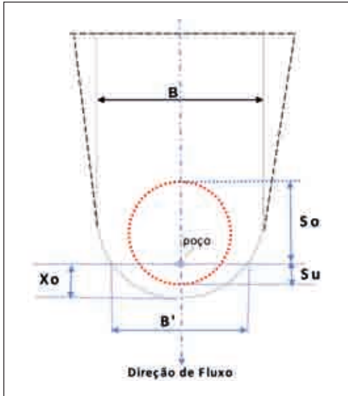
FIGURA C. Modelo de cálculo pelo método Wyssling
