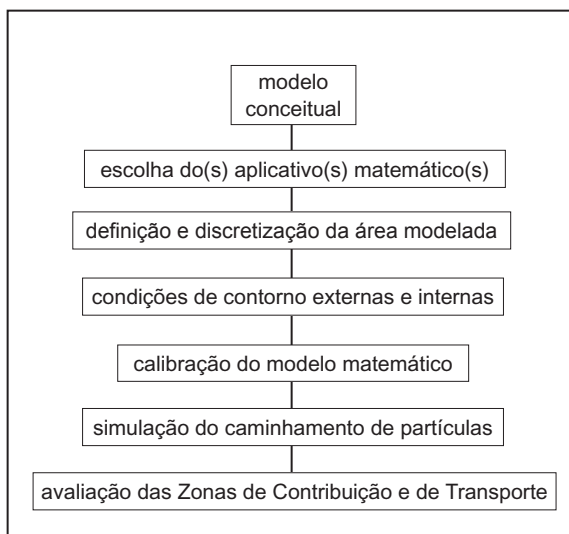
FIGURA D. Etapas de trabalho para a construção de um modelo matemático de fluxo da água subterrânea (Iritani 1999)
